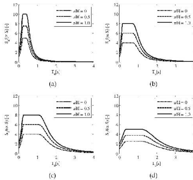
Figura C7.2.4 - Accelerazione massima, normalizzata rispetto ad aS, per i seguenti valori di T_d : (a) T_d = 0,3 s, (b) T_d = 0,6 s, (c) T_d = 0,9 s, (d) T_d = 1,2 s.
