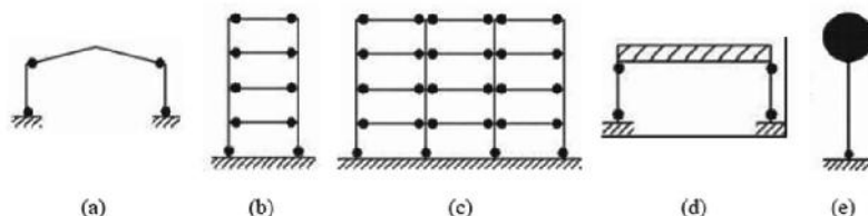
Figura C7.5.1 - Configurazioni dissipative di strutture intelaiate: disposizione delle cerniere plastiche, secondo le tipologie esposte nella tabella 7.3.11 del § 7.3.1 delle NTC
