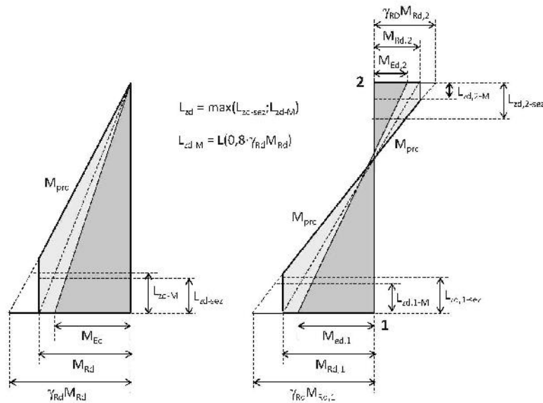
Figura C7.9.1 – Proiezione in capacità delle pile (schemi a mensola e a doppio incastro)
