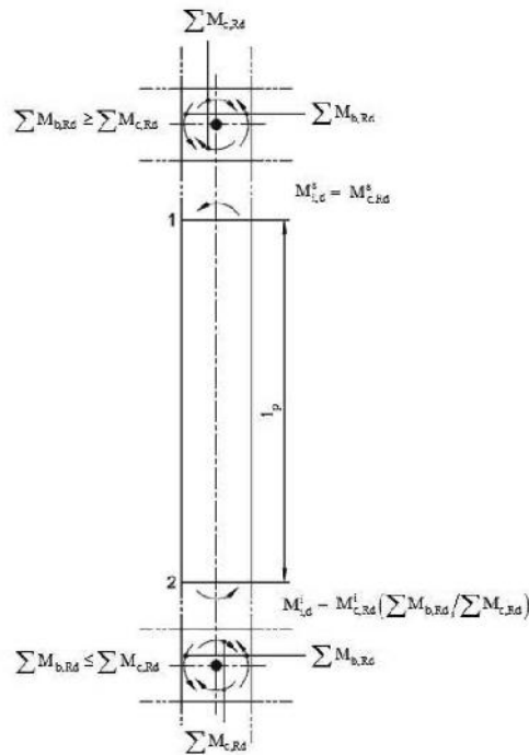
Figura C7.A.2 – Equilibrio dei momenti per il calcolo delle sollecitazioni di taglio di progetto V_{Ed} nei pilastri.
