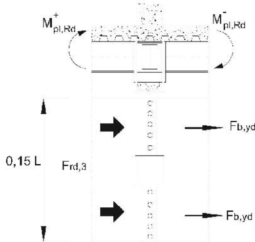
Figura C7.6.3 - Meccanismo 3 - Connettori a taglio sulle travi secondarie
