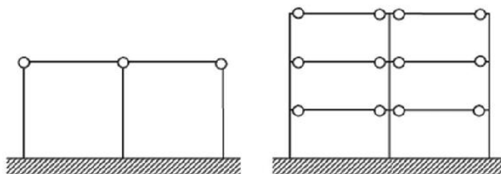
Figura C7.4.5 - Strutture con pilastri incastrati alla base ed orizzontalmente ad essi cernierati
