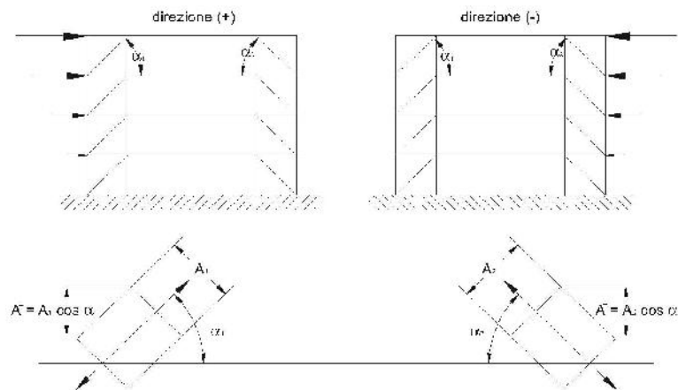
Figura C7.5.3 - Definizione dell'area delle sezioni dei controventi tesi, A^+ e A^- , da utilizzare nella formula C7.5.3
