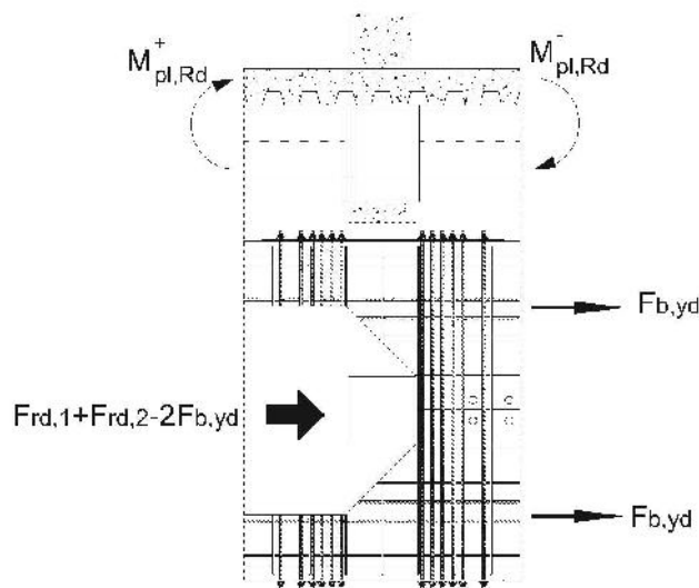
Figura C7.6.4 - Distribuzione e S.I.U. sotto azioni sismiche, delle massime resistenze agenti nella soletta del nodo.
