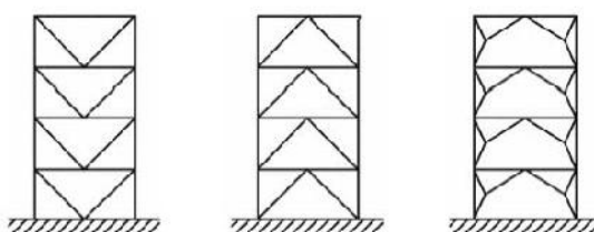
b2) Strutture con controventi concentrici a V
