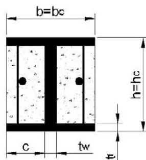
Fig. 7.6.1 - Rapporti dimensionali
